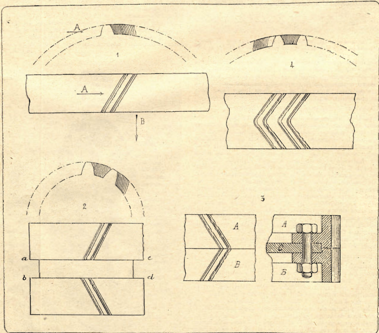
Fig. 5. — Ingranaggi elicoidali: 1, Reazioni su una dentatura dicoidale semplice: A, sforzo periferico per il movimento della ruota, B, spinta parallela all'albero; 2, Ingranaggi a cuspidi: a, b, c, d, gola per l'uscita dell'utensile; 3, Ingranaggi a cuspidi ottenuti unendo due corone su unico rapporto: A, B, corone a comuni denti elicoidali, C, supporto; 4, Ingranaggio a dentatura sinusoidale.
