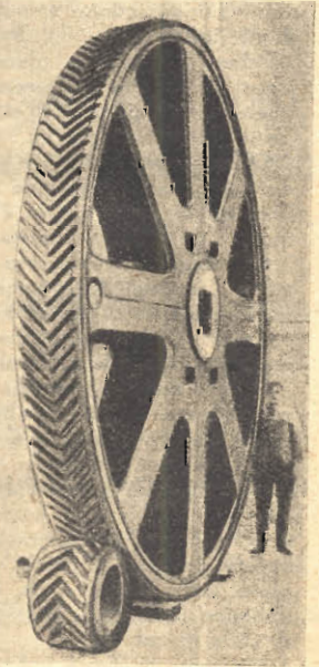
Fig. 2. — Ingranaggi a cuspidi tagliati in una corona unica.
