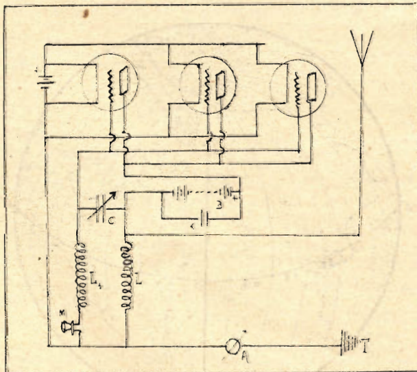
(v. fig.): aereo bifilare di 60 m.; batteria anodica di 200 a 300 volts; batteria filamento 6 volts; condensatore C, 0,002 mf.; A, milliamperometro termico; microfono a granelli; B, condensatore di batteria di un microfarad; L, cilindro coibente di 20 cm.
