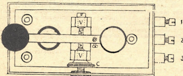
Proiezione orizzontale
