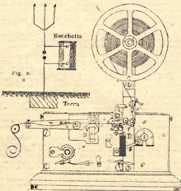
Fig. 2. — Macchina Morse.
